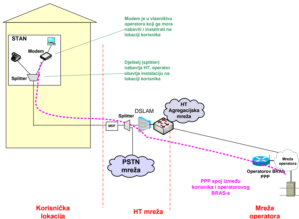
Slika 9. Način realizacije Veleprodajnog širokopojsnog pristupa za pružanje Internet usluge na DSLAM razini
