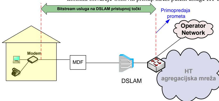
Slika 7. Veleprodajni širokopoljasni pristup za pružanje Internet usluge na DSLAM razini u slučaju kada krajnji korisnik ostvaruje Osnovni pristup mreži putem usluge HT-a
