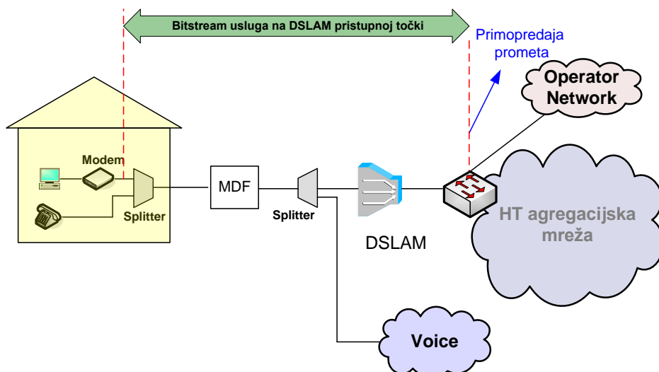
Slika 7. Veleprodajni širokopoljasni pristup za pružanje Internet usluge na DSLAM razini u slučaju kada krajnji korisnik ostvaruje Osnovni pristup mreži putem usluge HT-a
