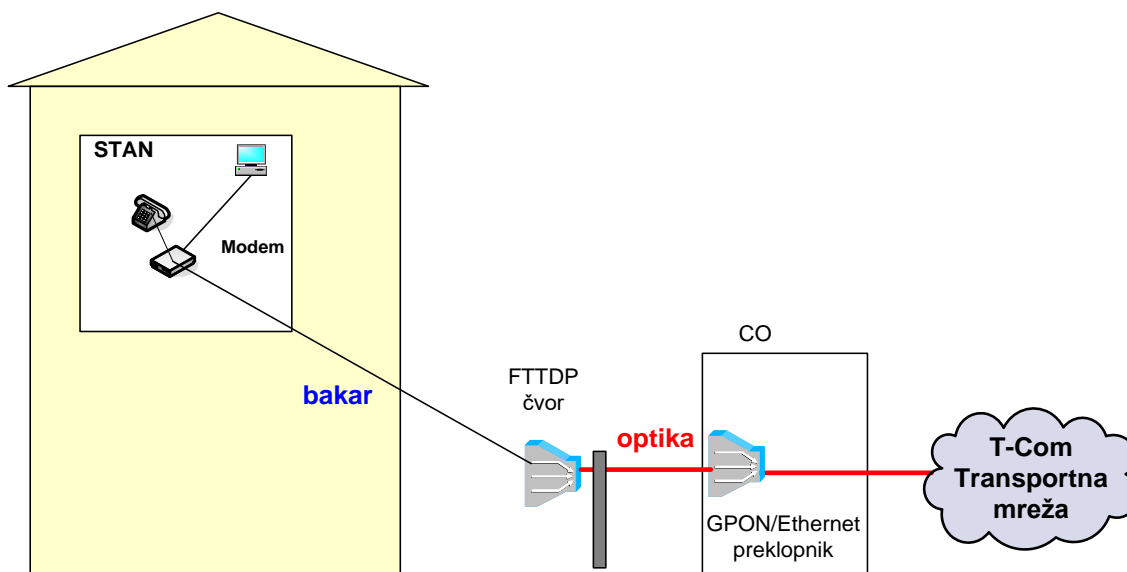
Slika 36. Način realizacije FTTDP koncepta sa VDSL17a tehnologijom u pristupnoj mreži
